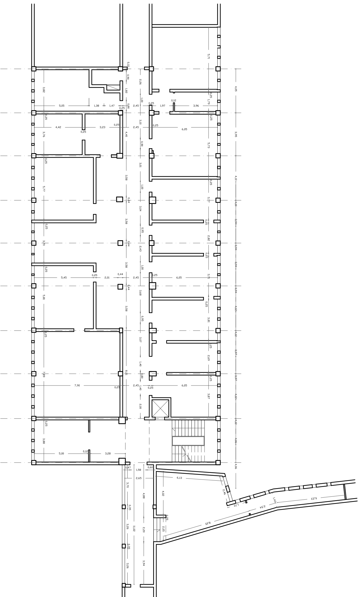
κάτοψη 2ου ορόφου κλίμακα 1:200
